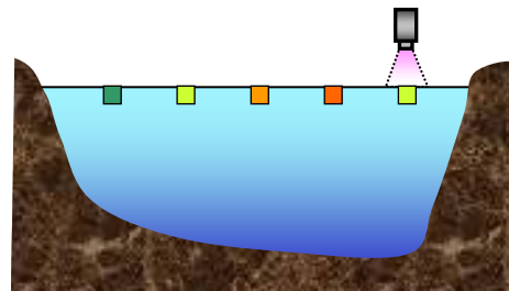
電波流速計
